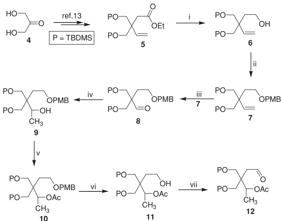
SCHEME 1 Synthesis of aldehyde intermediate 12 . Reagents: i) DIBAL-H, \text{CH}_2\text{Cl}_2 ; ii) PMBCl, NaH, THF; iii) \text{O}_3/\text{DMS} , \text{CH}_2\text{Cl}_2 ; iv) \text{CH}_3\text{MgBr} , THF; v) \text{Ac}_2\text{O} , pyridine; vi) DDQ, \text{CH}_2\text{Cl}_2 - \text{H}_2\text{O} ; vii) (\text{COCl})_2 , DMSO, \text{CH}_2\text{Cl}_2 , -78^{\circ}\text{C} .
